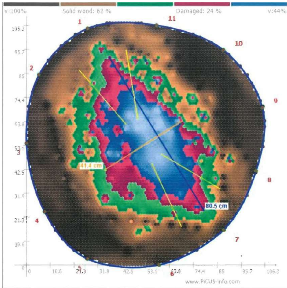
Obraz badania tomografem pnia na wys. 130 cm, grudzień 2018 r.
